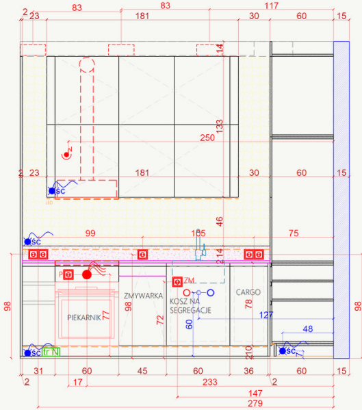
WIDOK D-D
