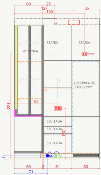
WIDOK A-A
